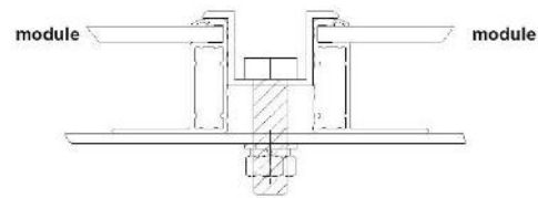
图B 组件夹具示例
