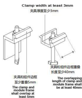
图A 组件夹具
